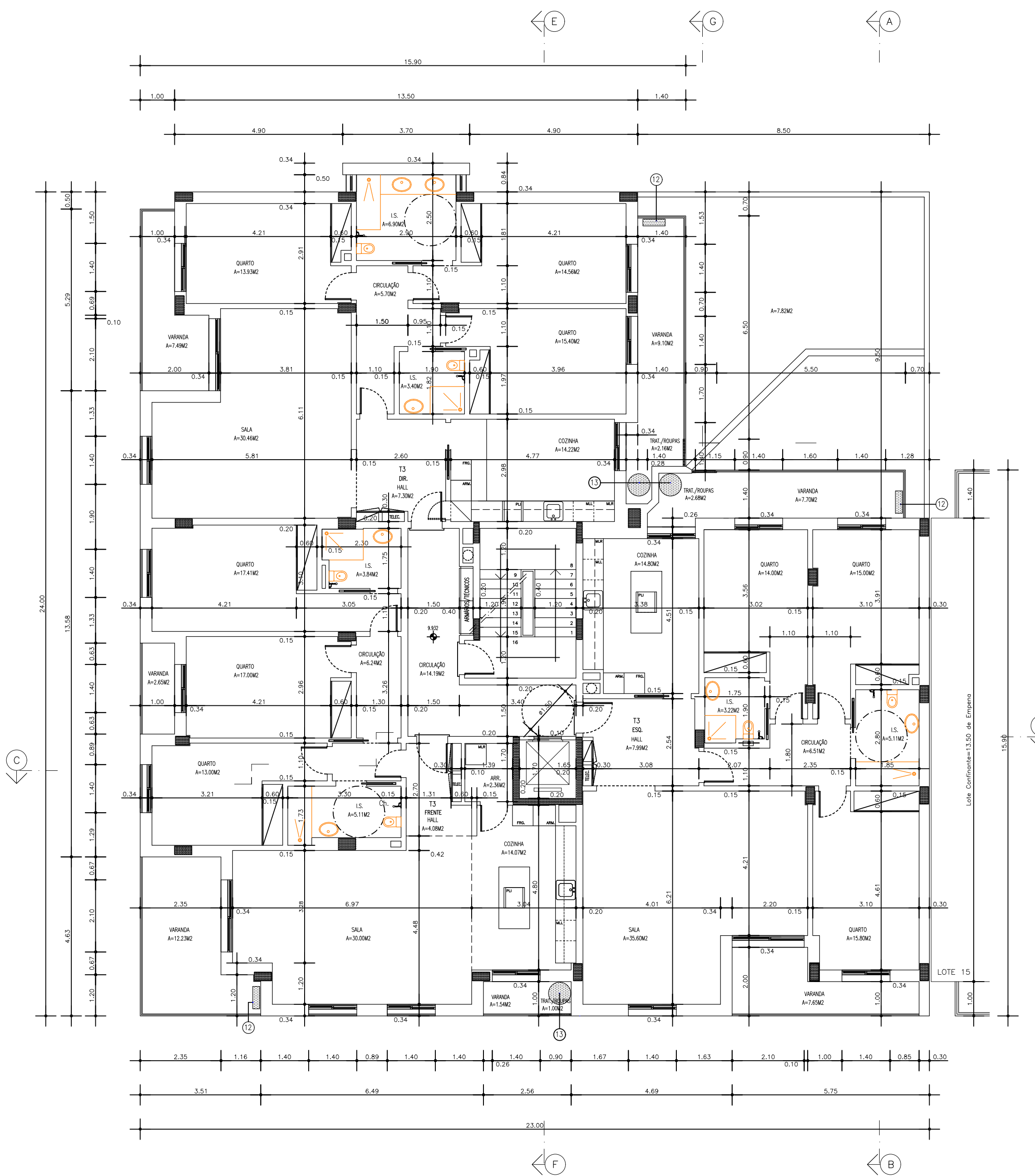
PLANTA PISO 1 ÁREA DO PISO = 441,57M 2 ÁREA VARANDAS = 50,582
